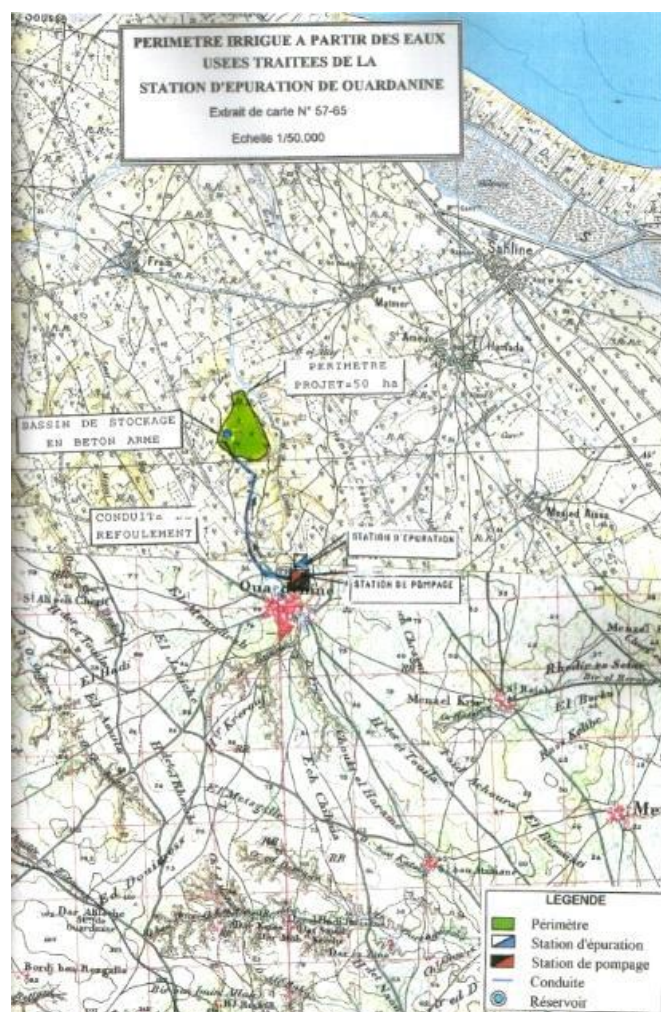
Figure 12: Plan du PI de Ouerdanine 25
