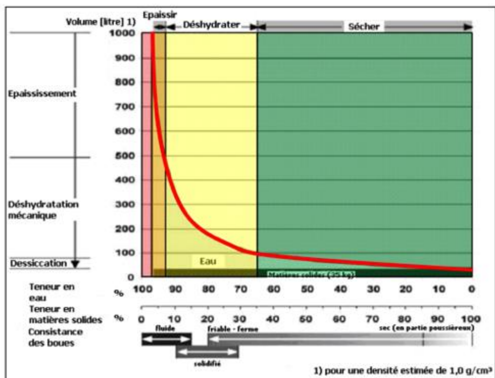
Figure 2. Evolution de la teneur en eau des boues suite aux trois procédés de traitement : épaissement, déshydratation et séchage
