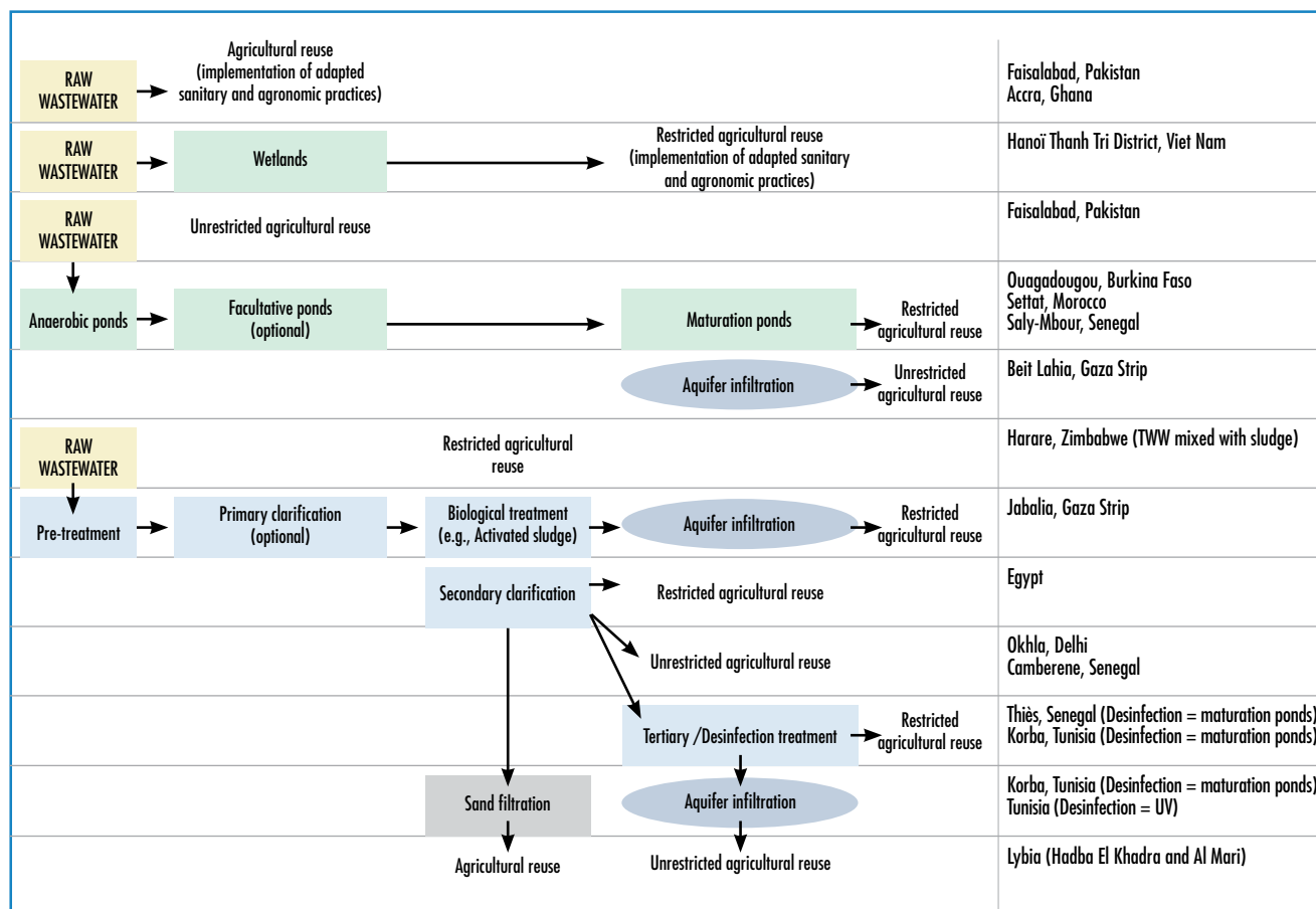
FIGURE 9 : Solutions de traitement mises en place dans certains pays en développement - Schéma Ecofilae
