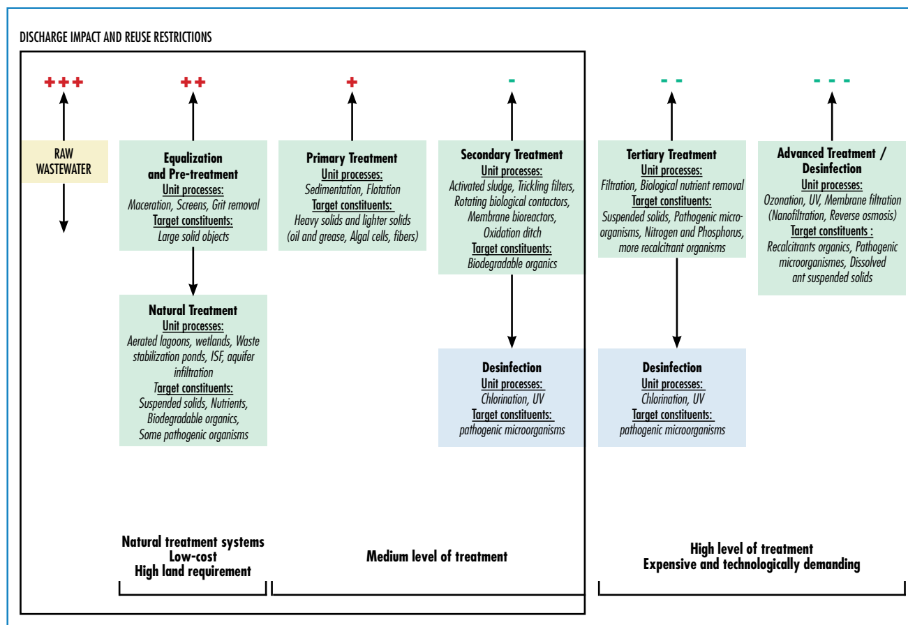
FIGURE 10 : Les procédés de traitement des eaux usées pour leur réutilisation - Schéma Ecofilae &amp; adaptation de Sharma and Sanghi, 2013
