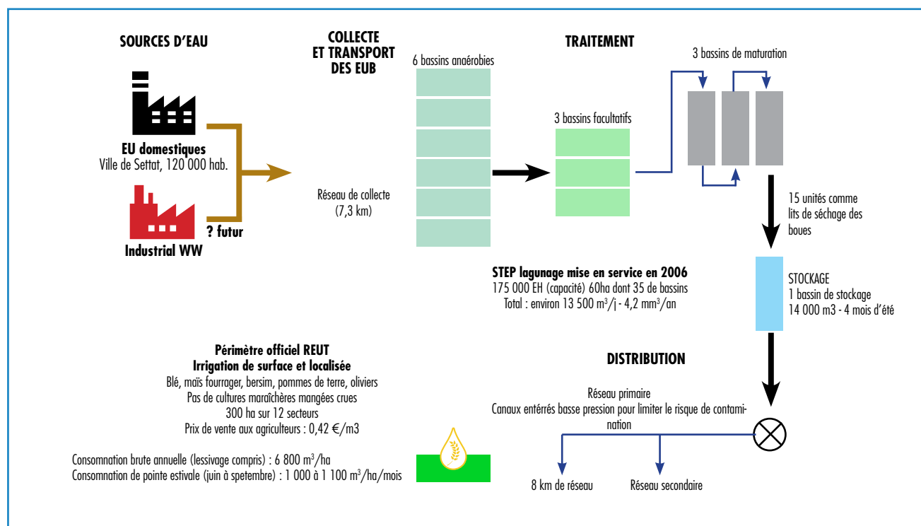
FIGURE 26 : La filière de réutilisation à Settât au Maroc - Schéma Ecofilae
