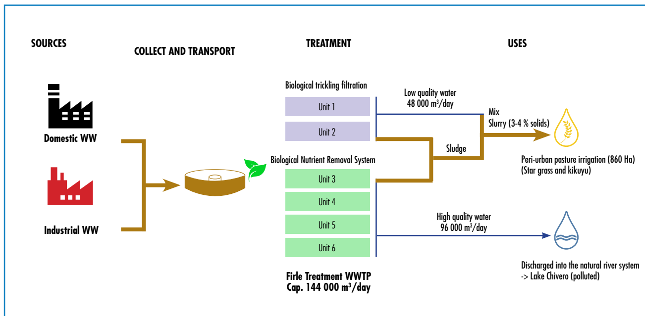
FIGURE 33 : La filière de réutilisation à Harare (Zimbabwe) - Schéma Ecofilae
