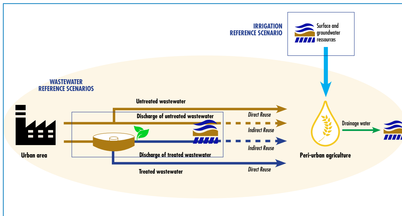
FIGURE 17 : Les interactions entre réutilisation des eaux usées et ressources en eau - Schéma Ecofilae
