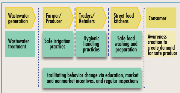
FIGURE 7 : L'approche multi-barrière pour la santé publique lorsque le traitement des eaux usées est limité – OMS 2006
