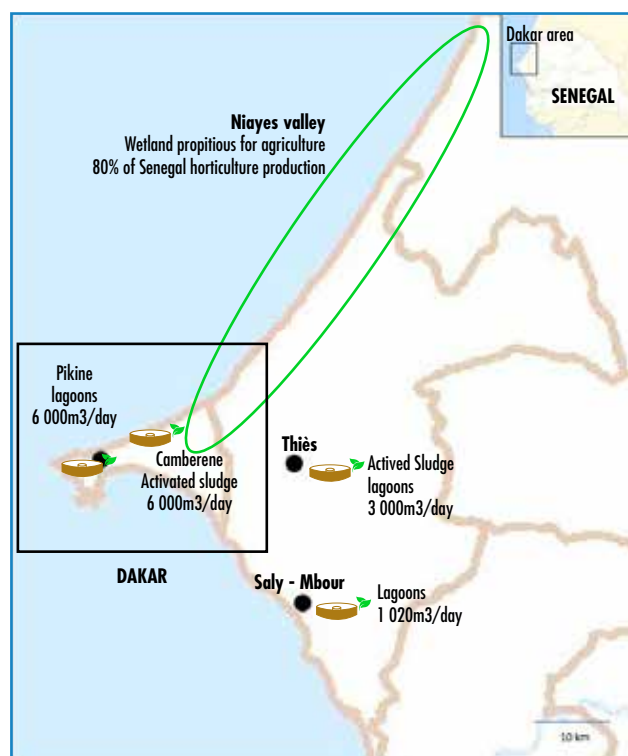
FIGURE 29 : Localisation d'expériences de réutilisation au Sénégal - Schéma Ecofilae
