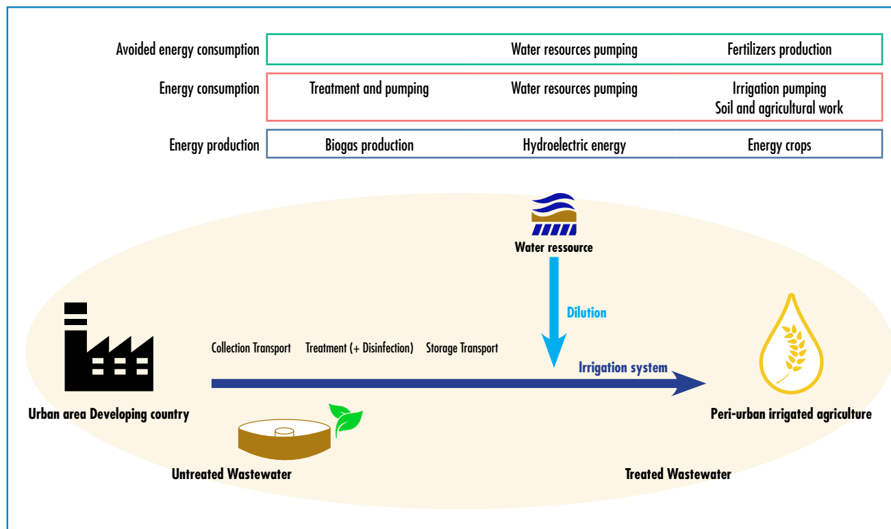
FIGURE 16 : Interactions entre réutilisation des eaux usées et énergie - Schéma Ecofilae
