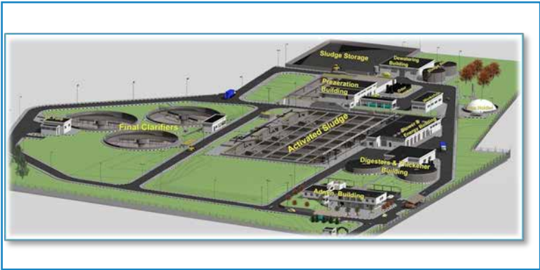
FIGURE 31 : Maquette de la station d’épuration de Jabaliya – ICID 2015
