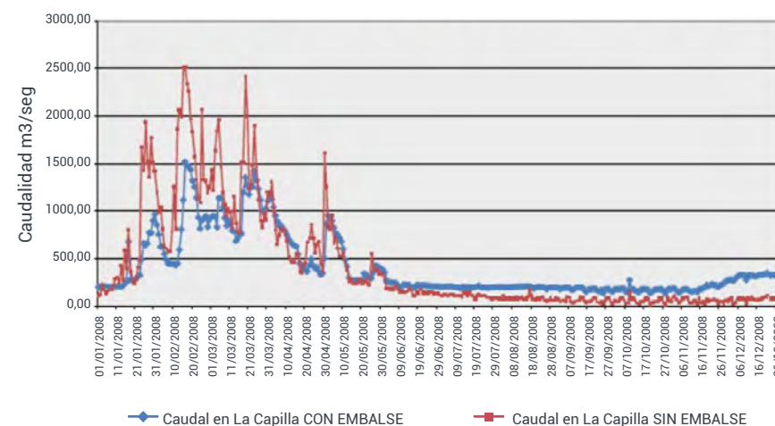
Gráfico 10: Efecto regulador del embalse Daule Peripa en el año 2008, en la estación La Capilla. Fuente: Hidronación.
